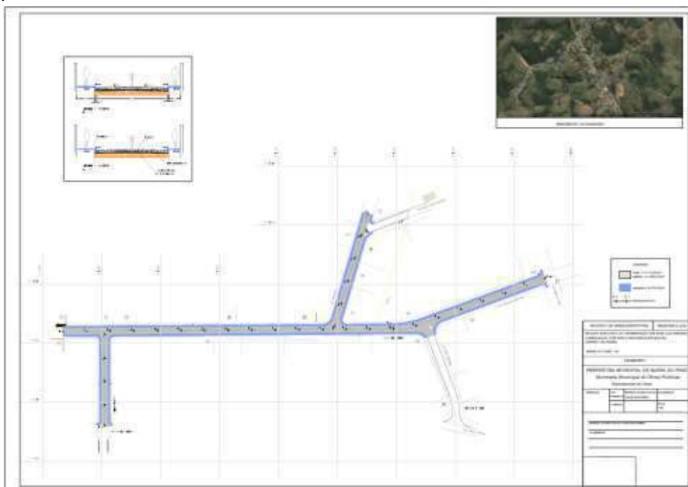
Figura 05: Projeto de Pavimentação – Ruas Luiz Pinheiro da Silva, Comandante José Faro e Negreiros
